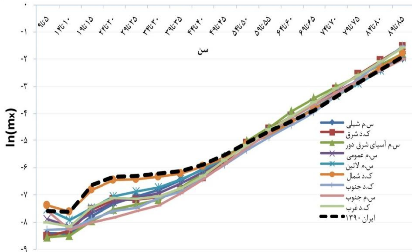
نمودار ۱. لگاریتم میزان‌های مرگ اختصاصی سن مردان ایران در ۱۳۹۰ و جداول عمر مدل‌های ۹ گانه
