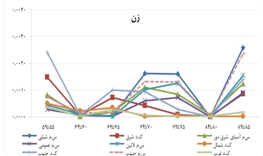
نمودار ۵. مربع باقیمانده‌ها بر حسب سن در رابطه لوچیت جدول عمر مشاهده شده ایران و جداول عمر الگو در سنین ۵۰ تا ۸۵ سالگی به تفکیک جنس
